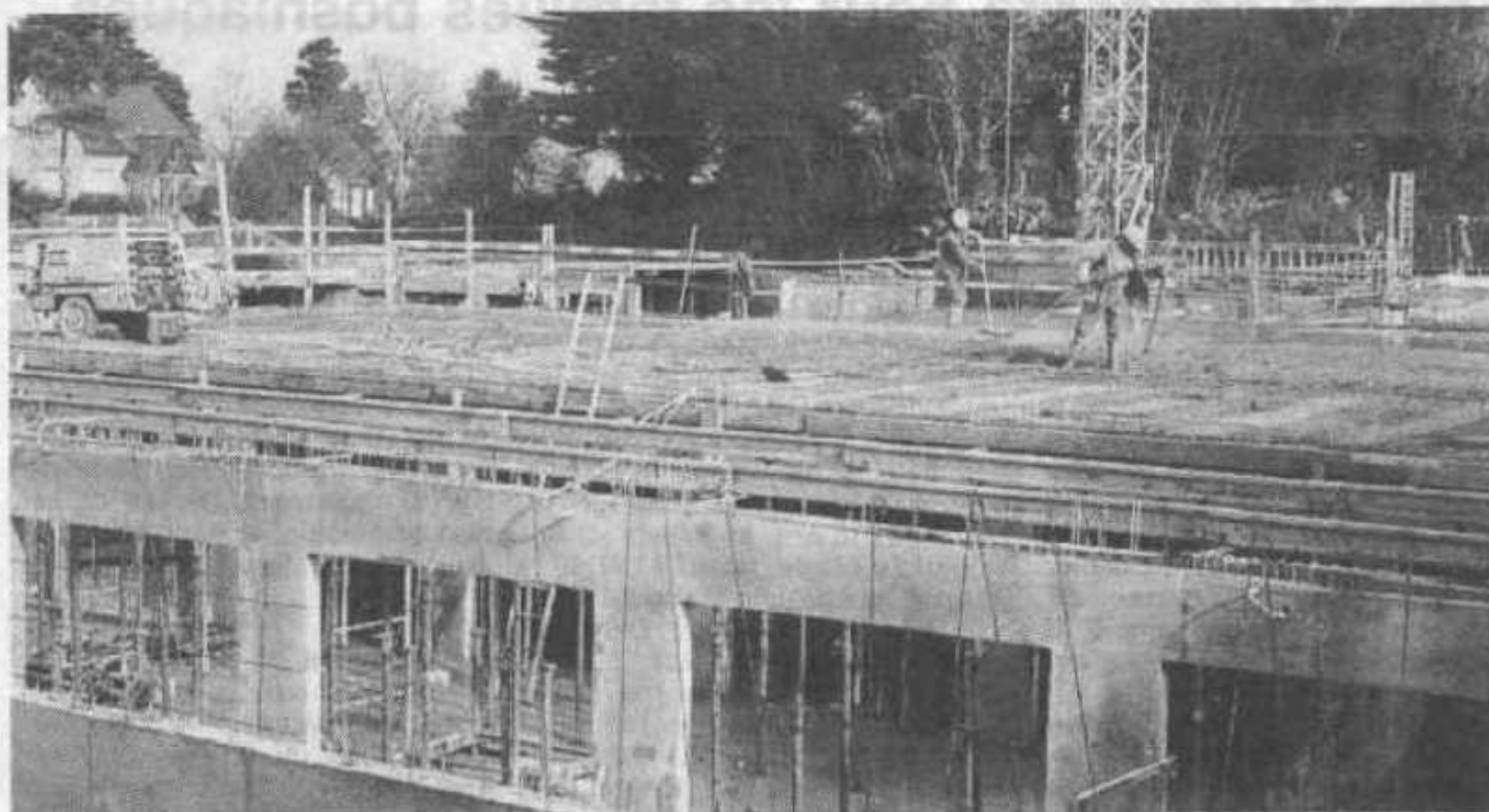
La seconde partie des garages souterrains est bien étayée. On coule actuellement la dalle de béton.
